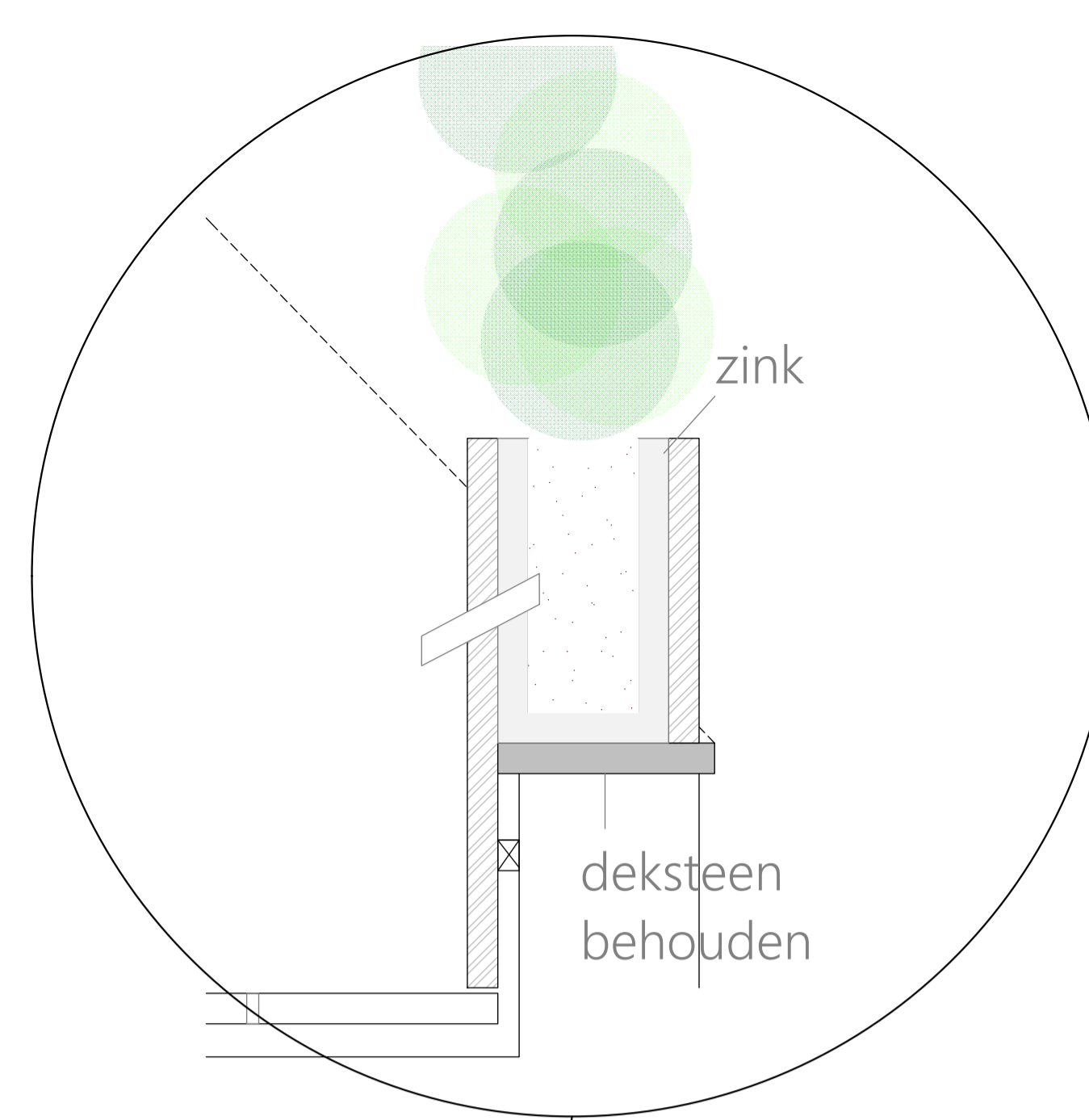
DOORSNEDE PLANTENBAK schaal 1/10
